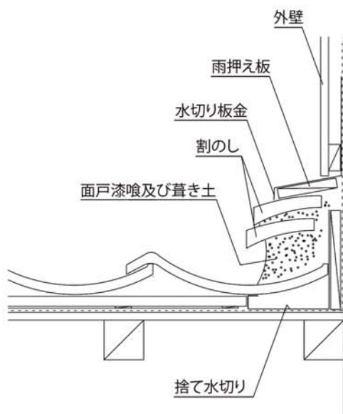
流れ壁際の納まり例 1
