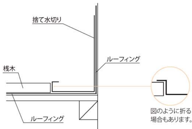
流れ壁際の納まり例 2
